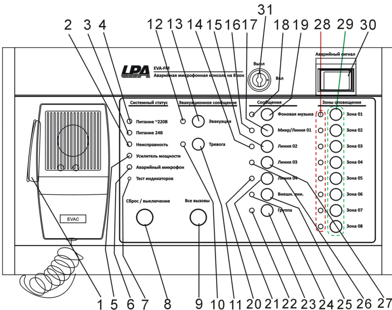
Рис. 3.2. Лицевая панель пожарной микрофонной консоли LPA-EVA-FM
