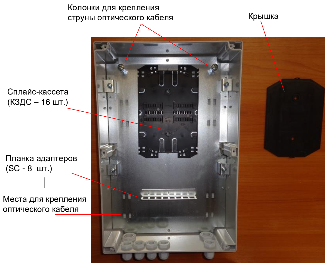
Рис. 2.4. Оптический кросс
