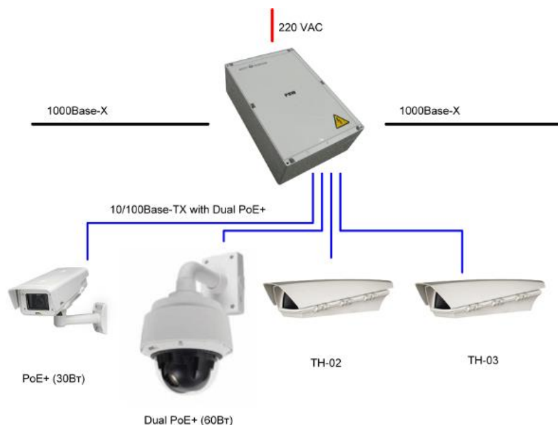
Рис. 1. Схема подключения PSW-2G+
