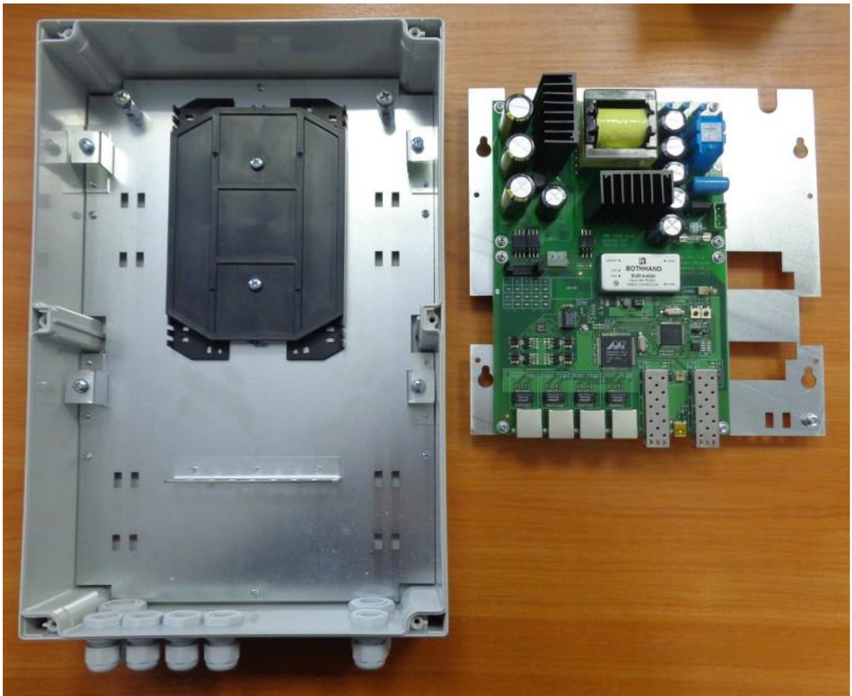
Рис. 2.1-3. PSW-2G+ - в разборе
