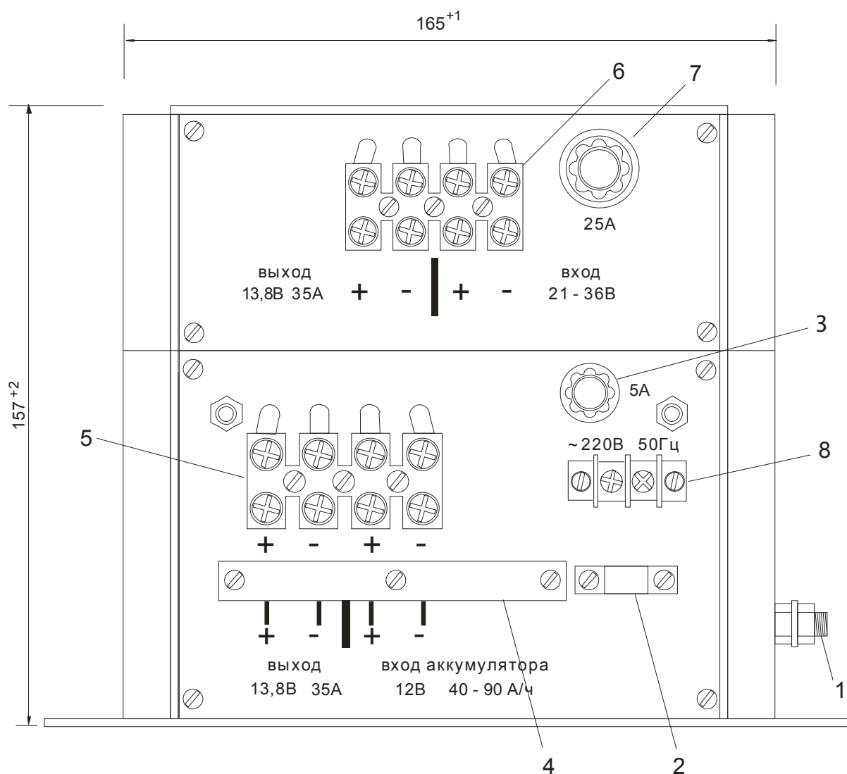
Рис. 2. Источник питания. Вид на заднюю панель, защитная крышка снята. 1-шпилька заземления. 2-скоба крепления сетевого кабеля. 3-держатель предохранителя источника питания ~220/12. 4-пластина фиксации проводов. 5-клеммы подключения нагрузки и АКБ. 6-клеммы подключения преобразователя напряжения к сети 24В. 7- держатель предохранителя преобразователя напряжения 24/12. 8-клеммы подключения источника питания к сети ~220В.
