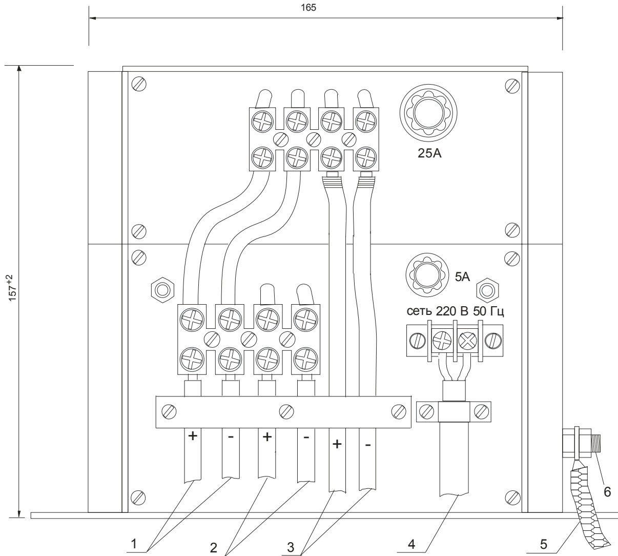
Рис. 3. Источник питания. Вид на заднюю панель, защитная крышка снята. Схема подключения.
